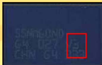
捺印文字欠け不良品 (目視で検出)
